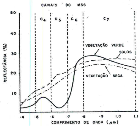
Fig. 2. Curvas de comportamento espectral (médias) para solos, vegetação verde e vegetação seca na faixa de sensibilidade do MSS do LANDSAT. FONTE: McDaniel and Hass (1982).
